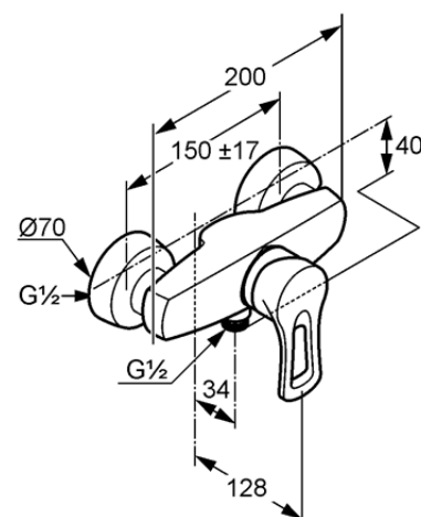
Размеры
